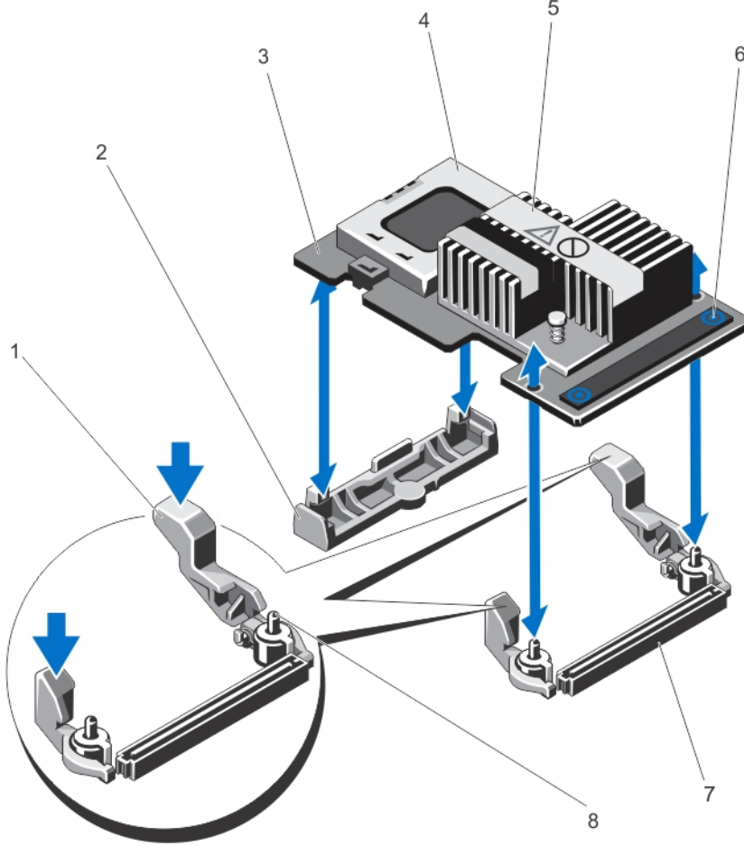
Rakam 3. PERC Mini Monolithic Denetleyicisinin Çıkarılması ve Takılması
